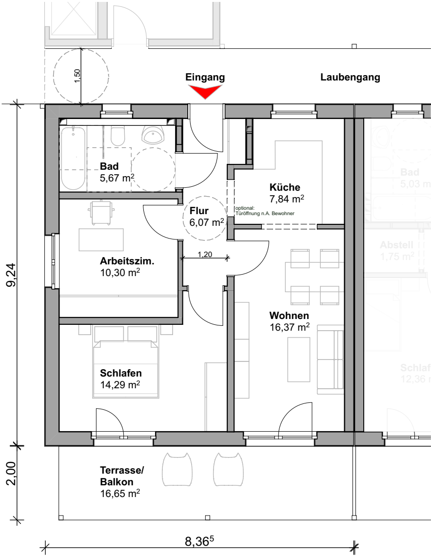
Grundriss
