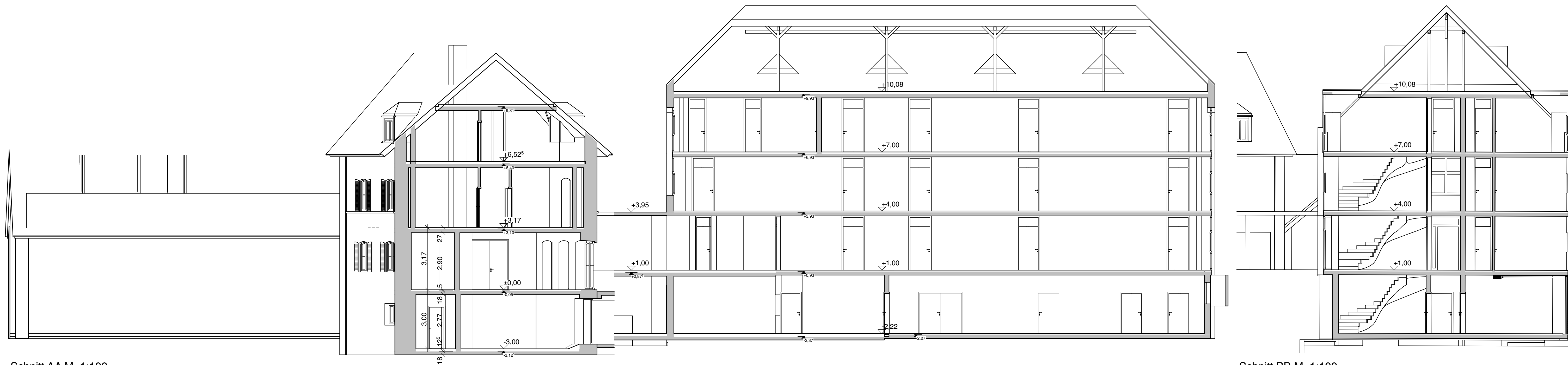
Schnitt AA M. 1:100
