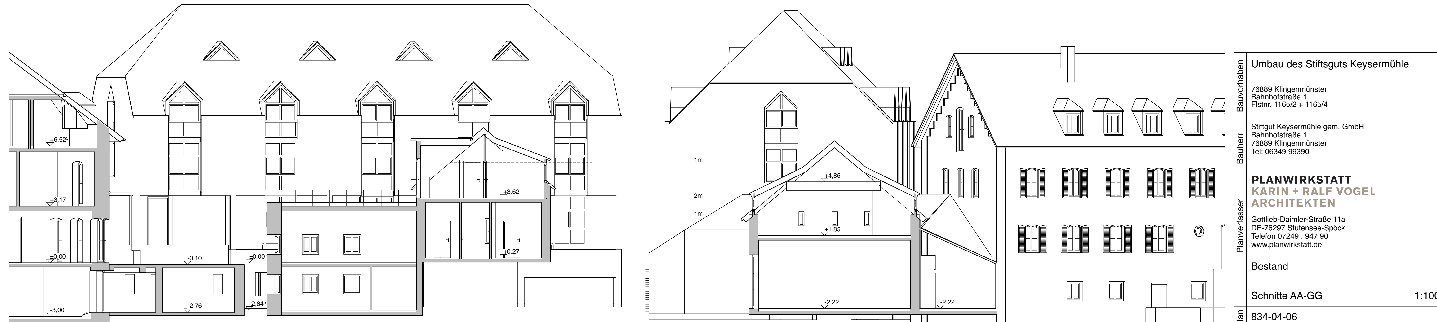
Schnitt FF M. 1:100
