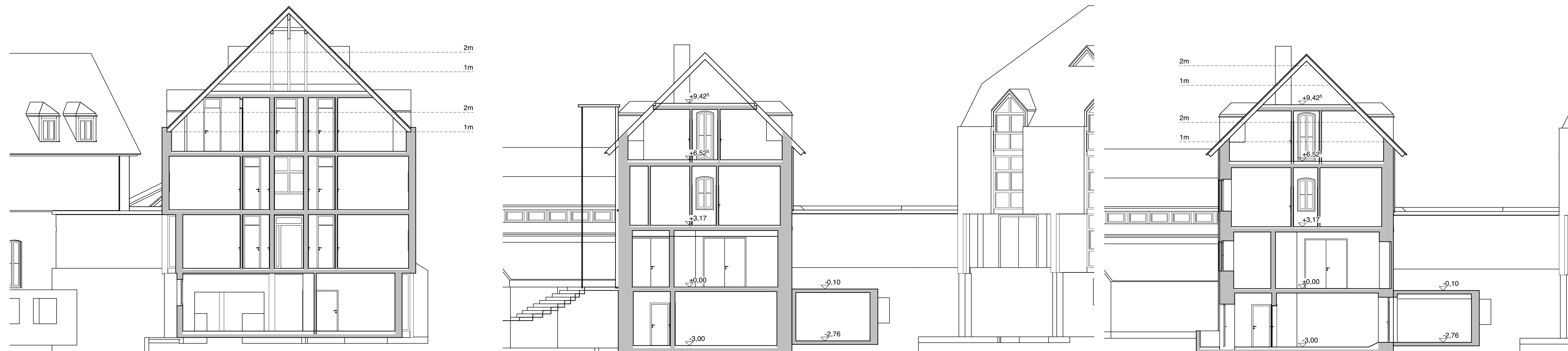
Schnitt CC M. 1:100
