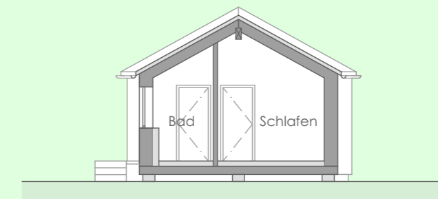
Schnitt CC
